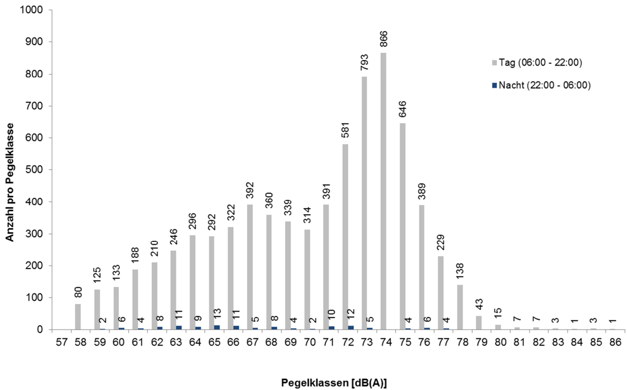
Häufigkeitsverteilung der Maximalpegel (korrelierte Fluggeräusche) Hégenheim 14/11/2012 – 28/02/2013
